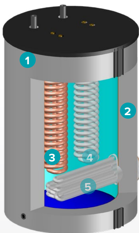
Abb.: Schnittmodell F-PD 250 (Solar)
