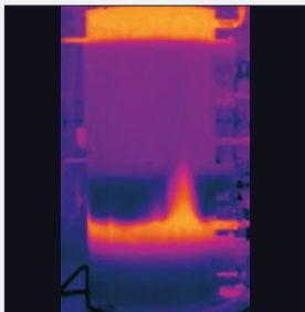
Hohe Warmwasserleistung durch die Nachschichtung von der unten in die obere Pufferzone.
